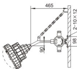
壁式(B1)30°
