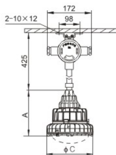
吊杆式(G)
