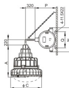
壁式(B2)90°
