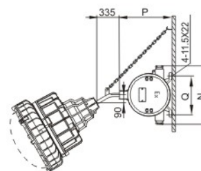
壁式(B1)30°
