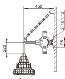
壁式(B2)90°
