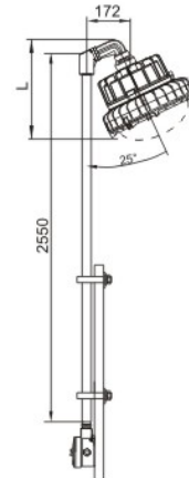
护栏式(h2)
